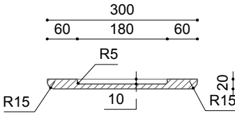
SECTION CUT A-A.
