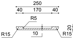
SECTION CUT A-A.
