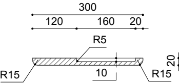
SECTION CUT A-A.
